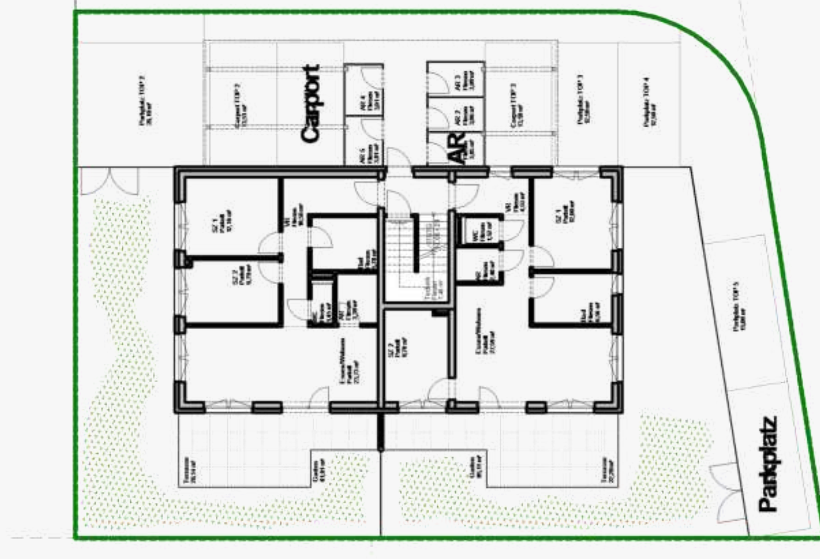
Übersicht Erdgeschoß
