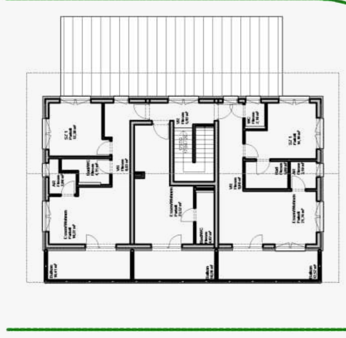
Übersicht Obergeschoß
