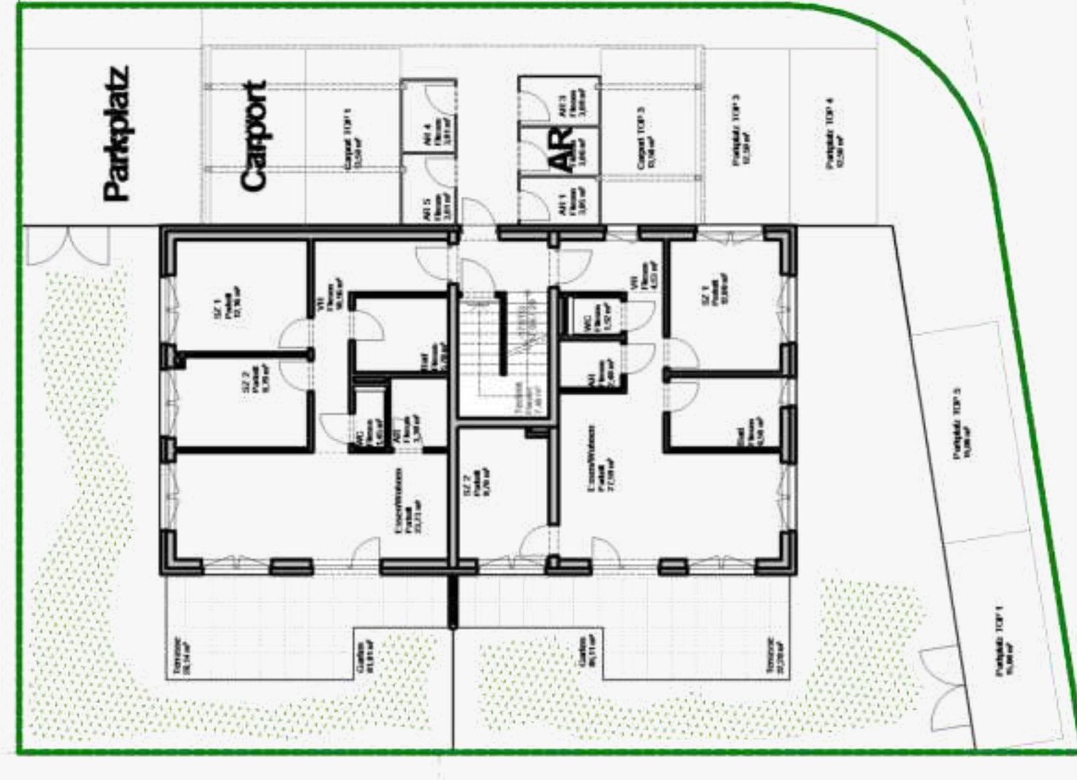
Übersicht Erdgeschoss
